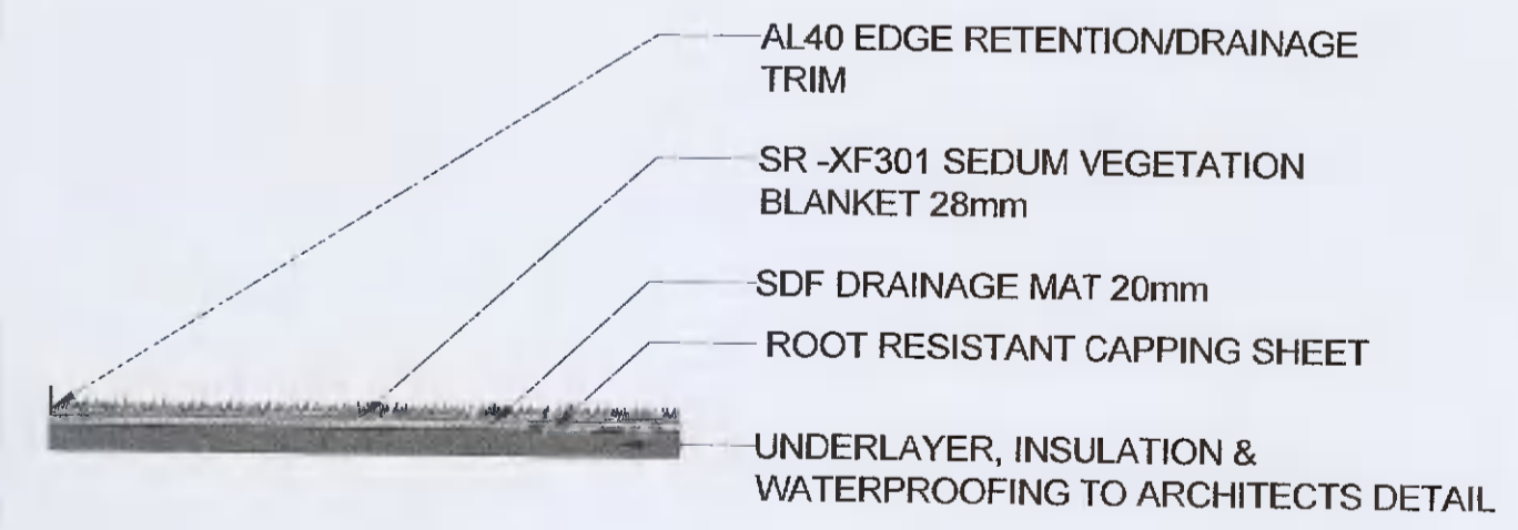
02 SEDUM ROOF 7200 Scale 1:20@A1
