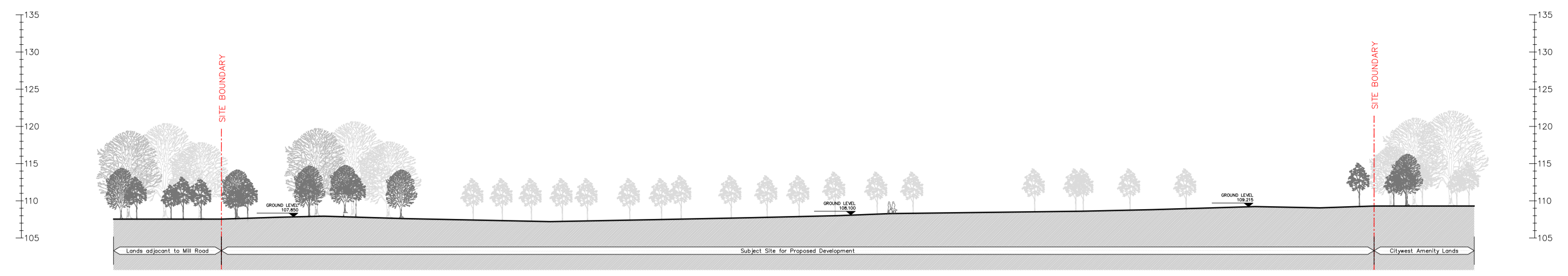
01 Existing Site Section DD EX 203 1:500
