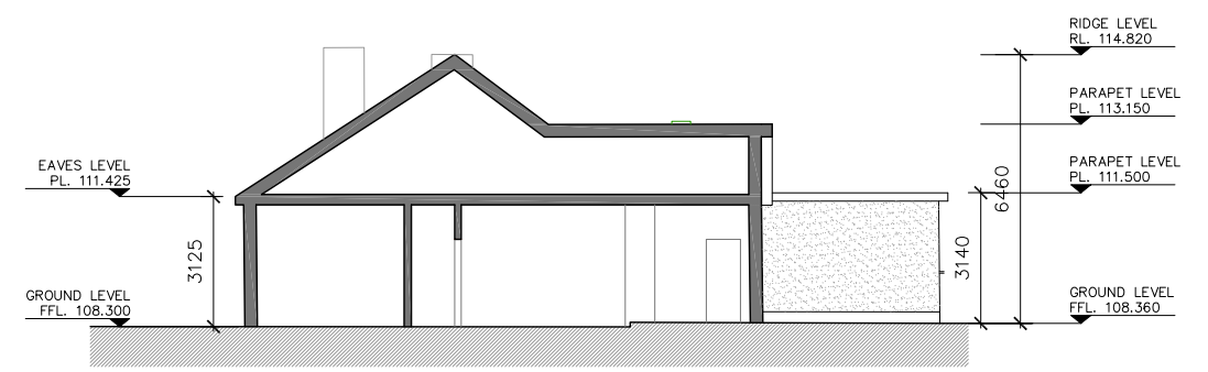
06 Section A-A EX-100 1:200
