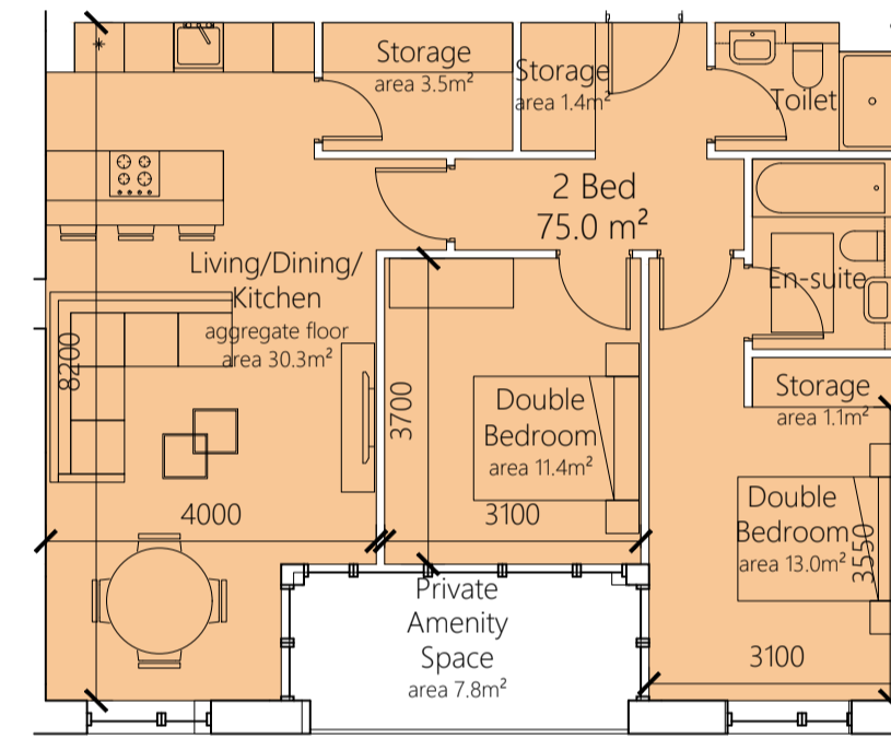
2 BED 4 PERSON i.e. D.1.9 D.2.17 D.3.25 D.4.32 TYPE: 2B4P O1 AREA: 75 m 2
