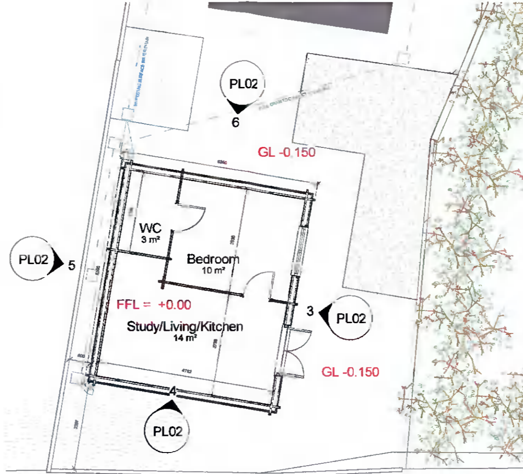
Floor Plan 1 : 100
