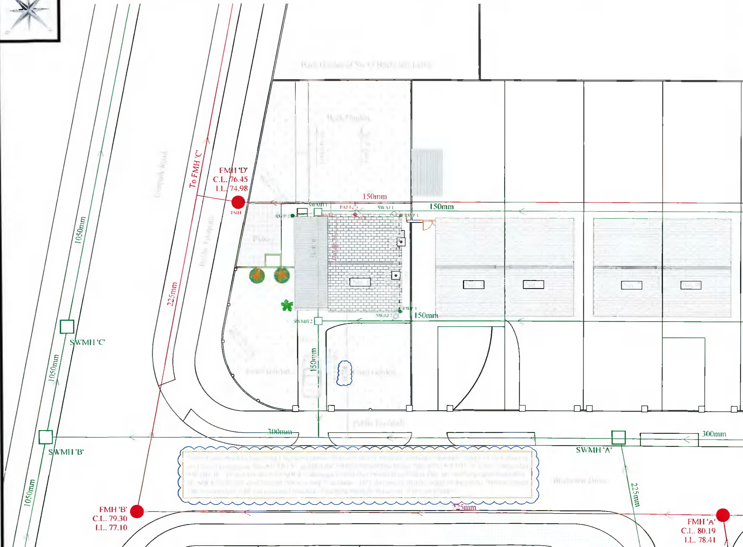
31 Existing Drainage Plan Scale: 1:200
