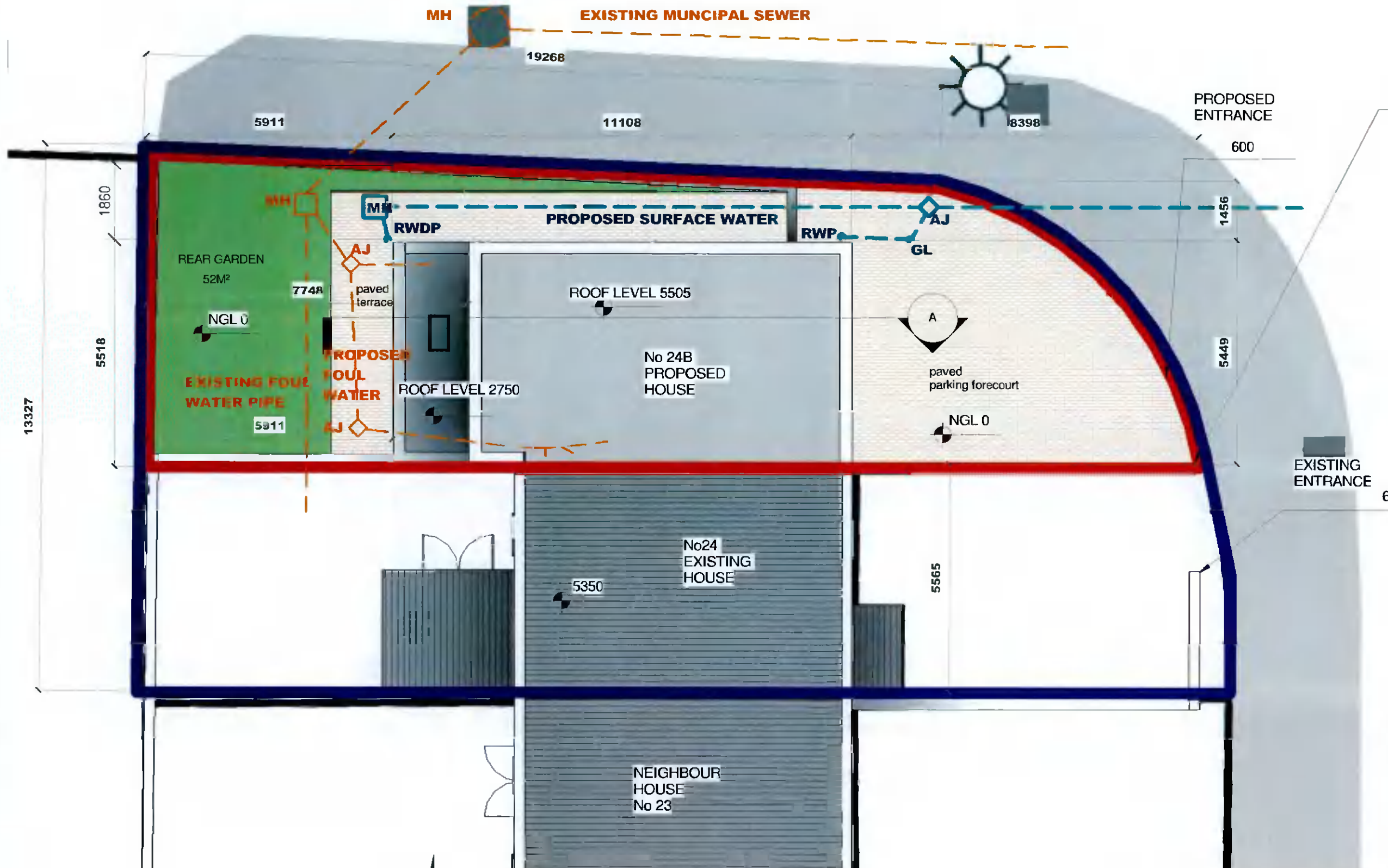
1 SITE PLAN 1 : 100
