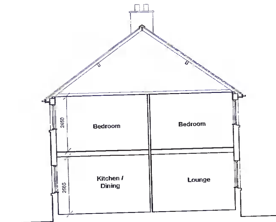
SECTION Scale: 1/100
