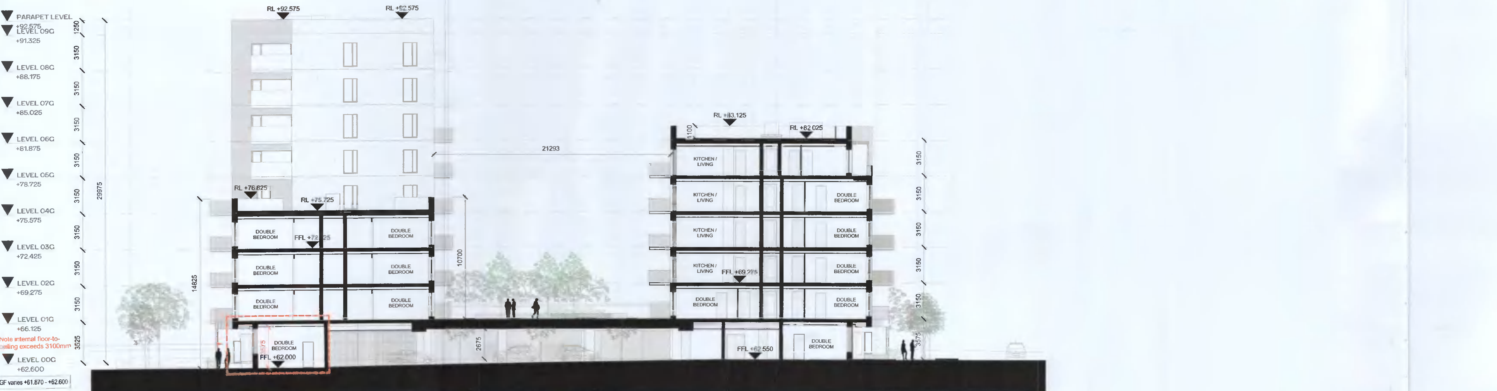
3 GA - SECTION - CC 1 : 200
