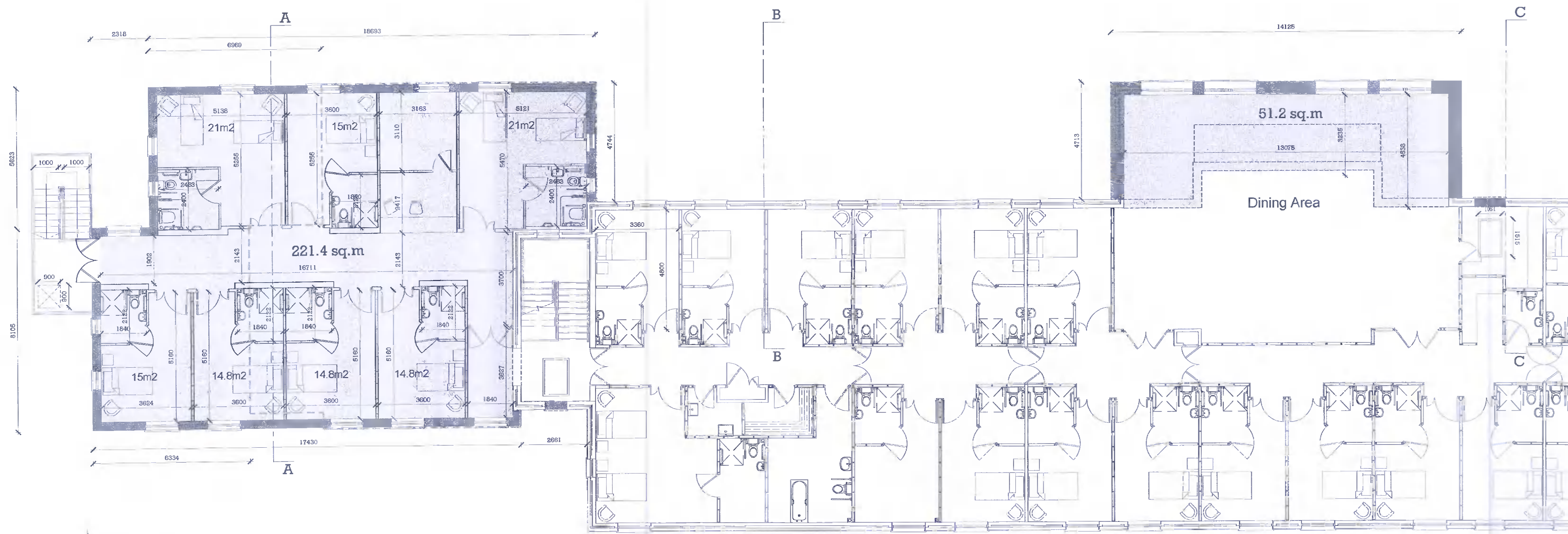
03 FIRST FLOOR A SCALE: 1:100
