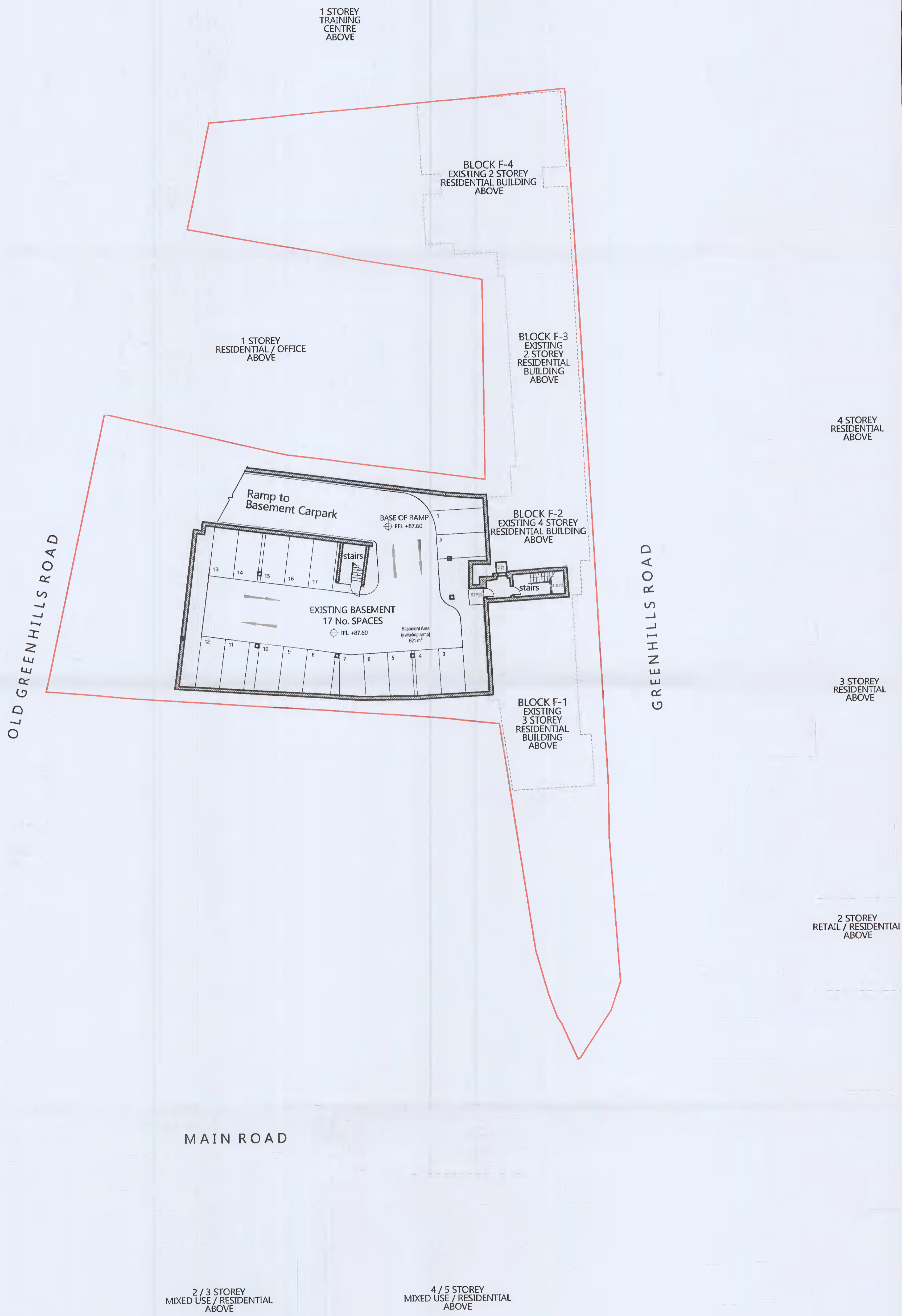
1 EXISTING BASEMENT PLAN AI-200 Scale: 1:200
