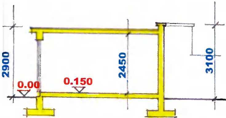
section a.a 1:100.
