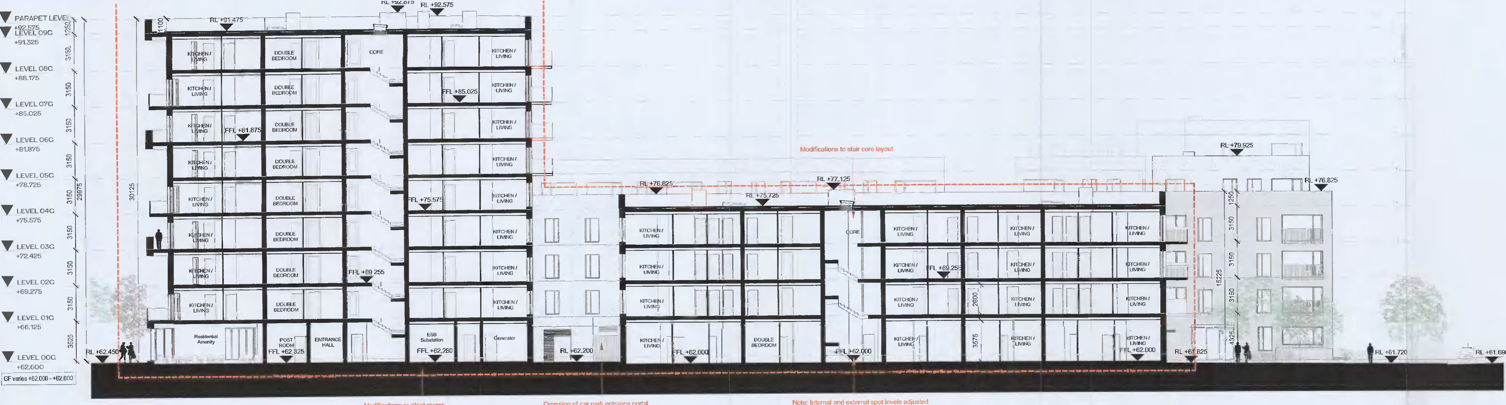
1 GA - SECTION - AA 1 : 200
