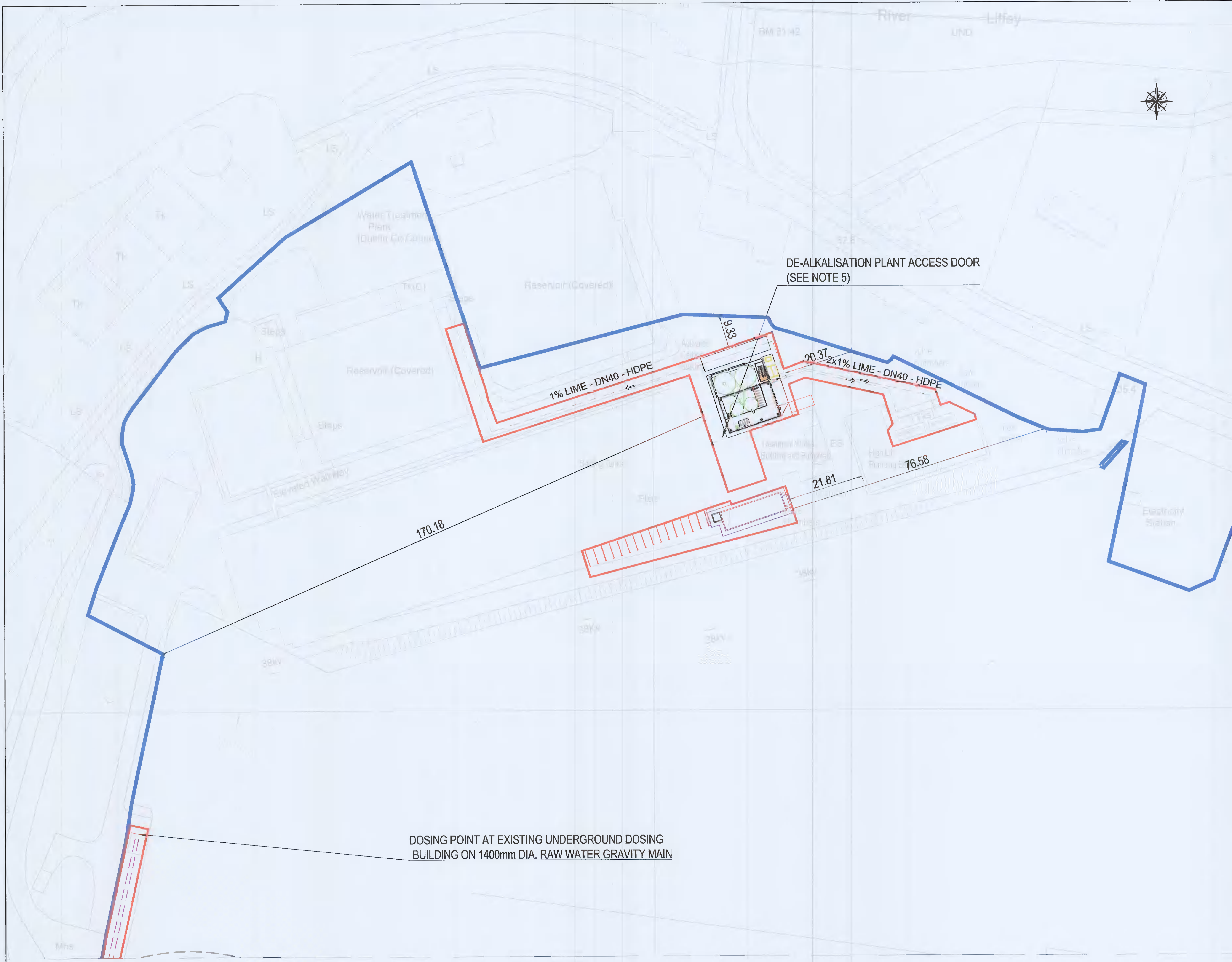
1 SITE LAYOUT (PART 1) 1 : 500
