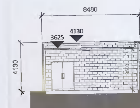
17 03023 Pumphouse - Section 1 : 200
