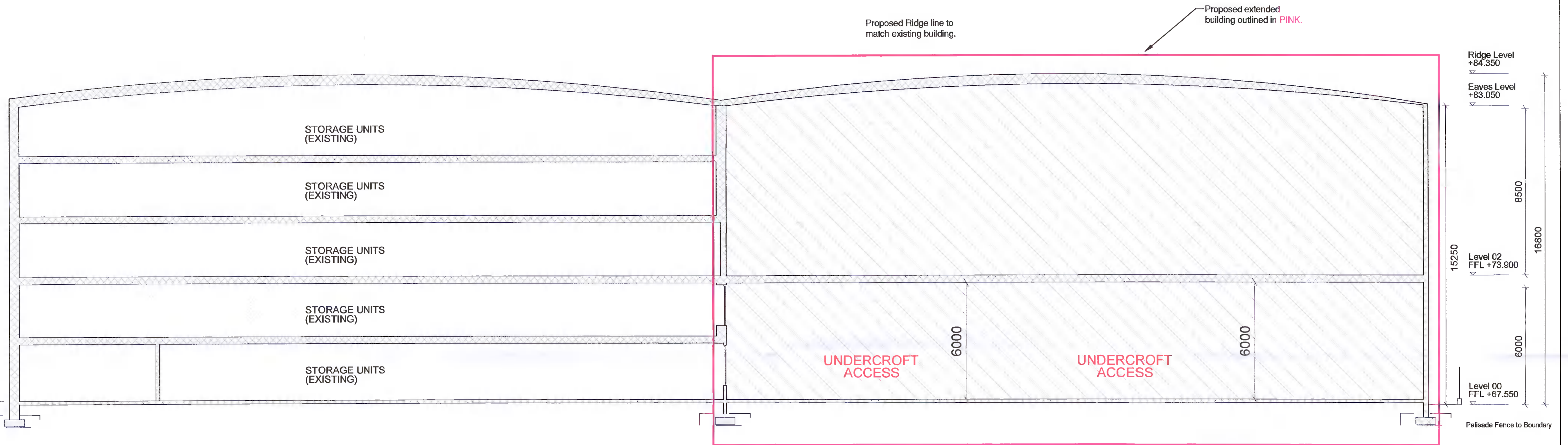
01 Section A-A A-A 1:100
