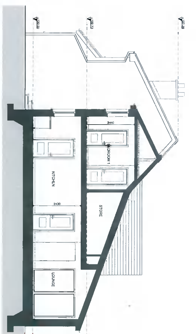
EXISTING SECTION A-A SCALE 1:50 @ A1, 1:100 @ A3
