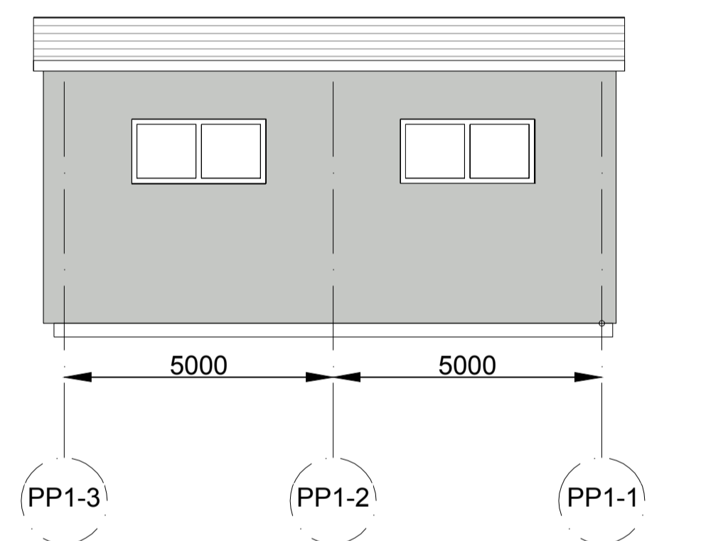
Elevation S4
