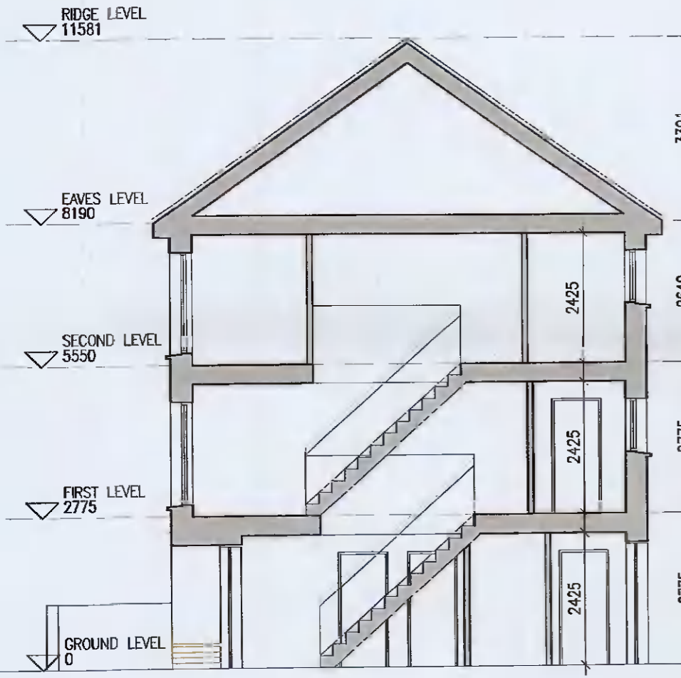
09 Section A-A 1:100@A1
