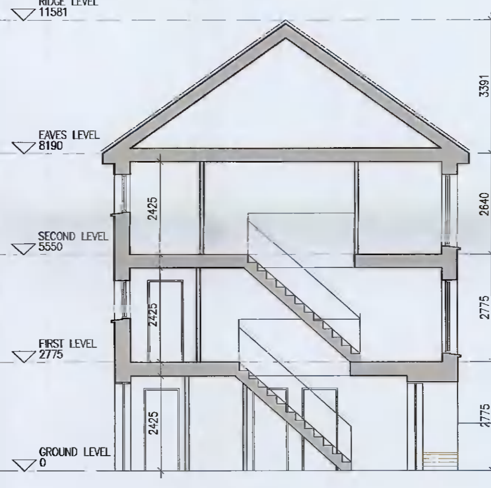
12 Section A-A 1:100@A1
